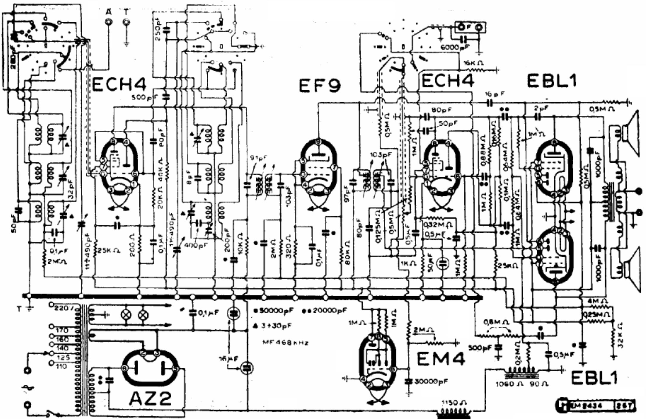
PHILIPS RADIO - « DI 670/A » « DI 680/A »
